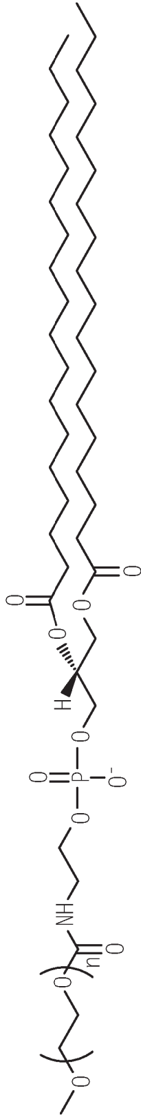
PEG-DSPE
